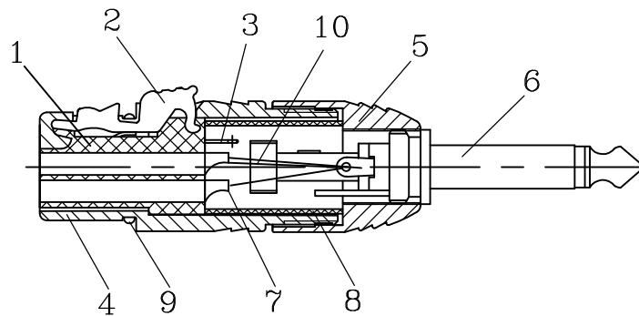
A-A SECTION
