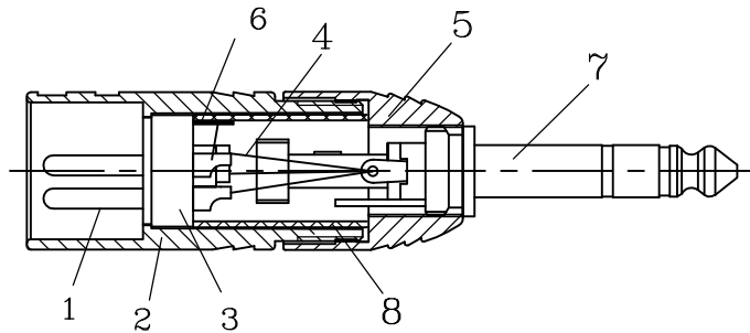
A-A SECTION
