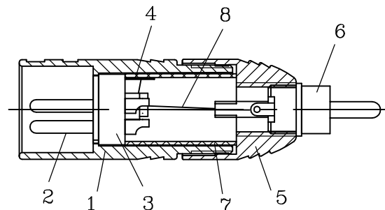
A-A SECTION
