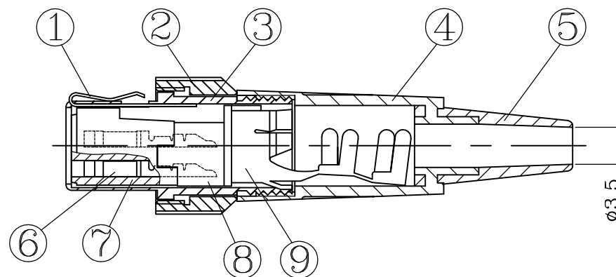
A-A SECTION
