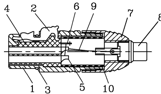
A-A SECTION
