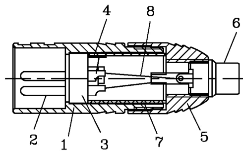
A-A SECTION
